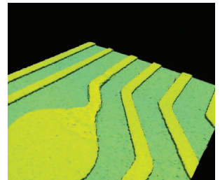
斷路 3D 成形後
