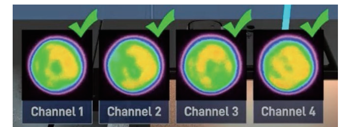
内置摄像机可验证四个钻孔通道的光束品质
