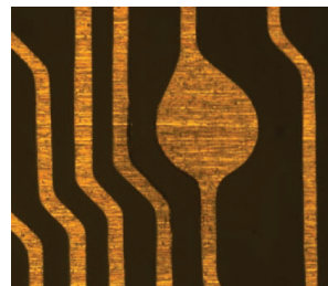
短路成形后 白光图像
