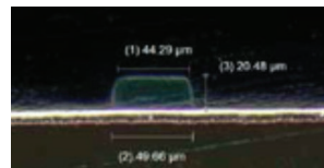
50µm 防焊桥， 铜上 20µm 防焊厚度
